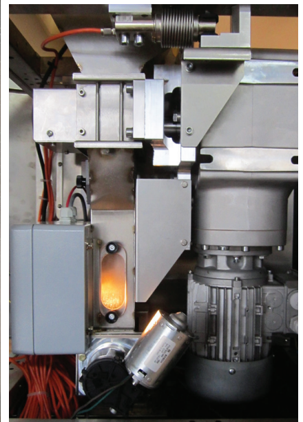
Abb.3: Innenansicht BA-T 300
